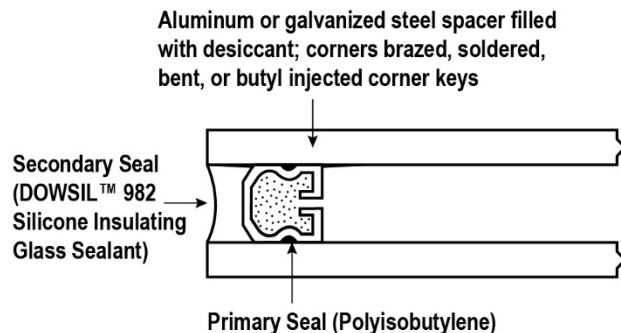
Figura 1: Vedação dupla
